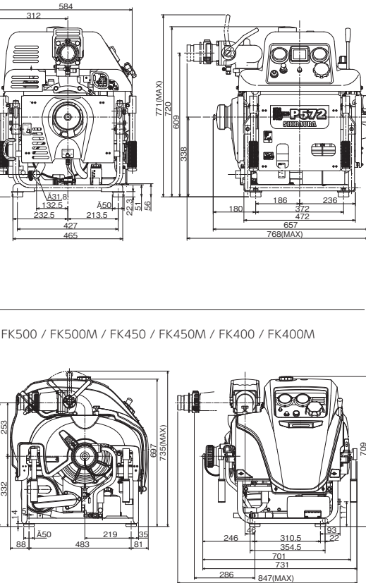
■寸法表 P572S
