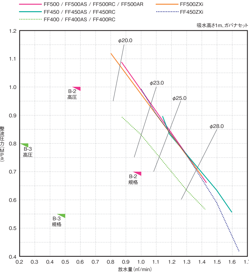
■性能曲線 FF500 / FF500AS / FF500RC / FF500AR / FF450 / FF450AS / FF450RC / FF400 / FF400AS / FF400RC / FF500ZXi / FF450ZXi
