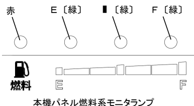
本機パネル燃料系モニタランプ
