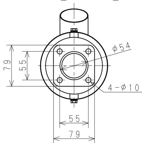
A 矢視
