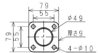
エキゾーストフレキ 接続口詳細 (1/4)
