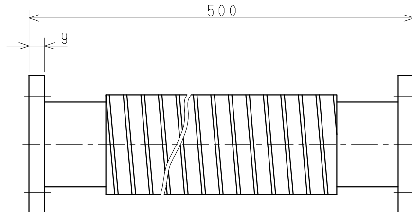
エキゾーストフレキ 1個
