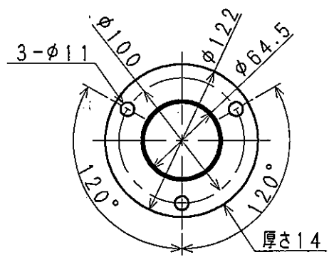
エンジン排気口詳細 (1/3)
