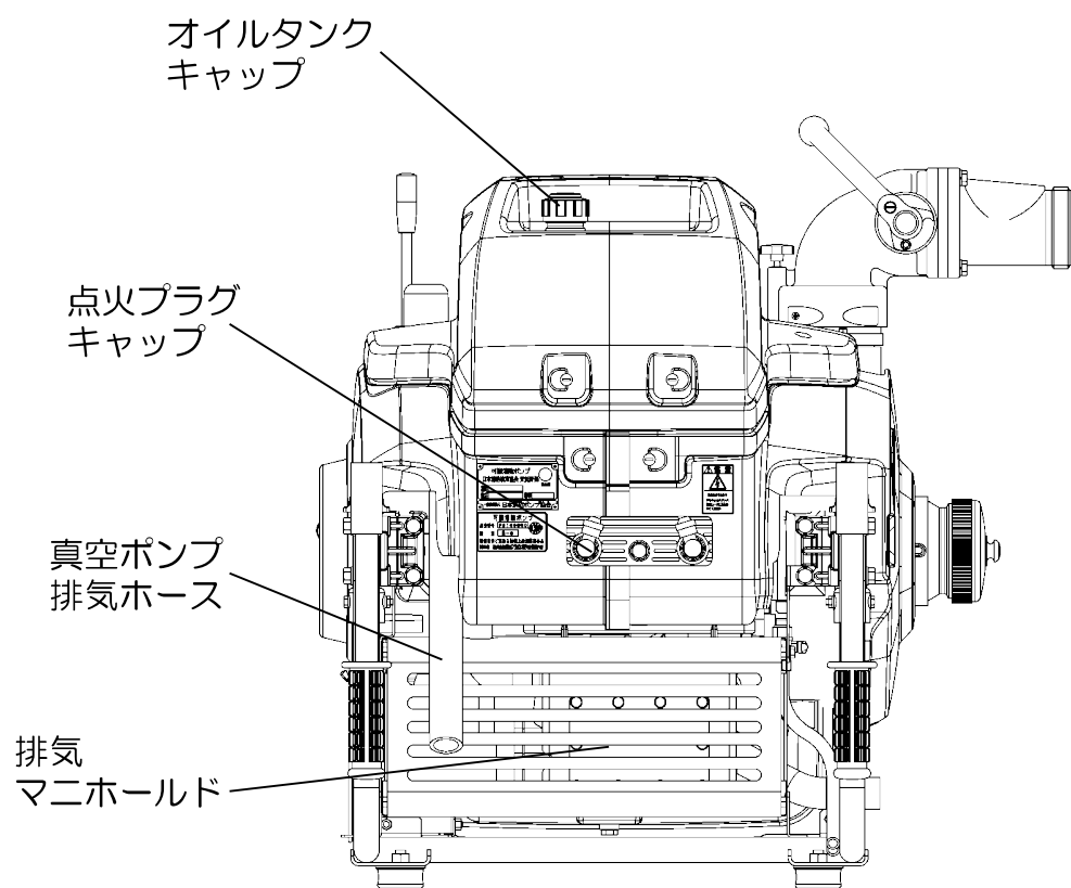
【反操作側】
