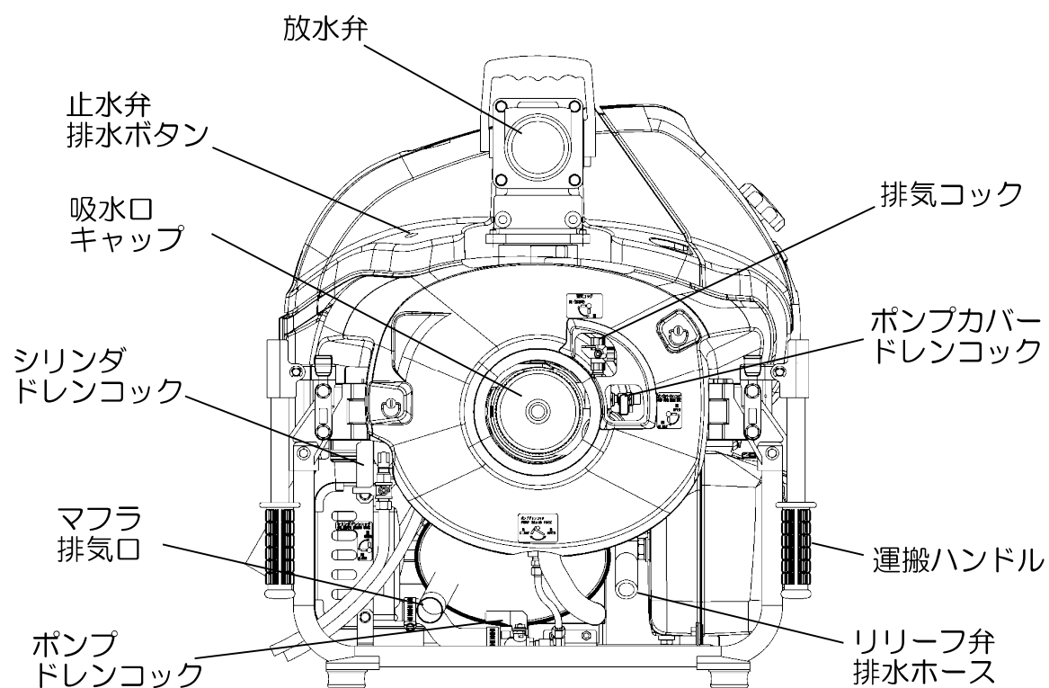
【ポンプ側】
