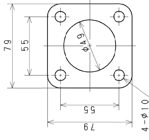
相フランジ (SS400) 2個
