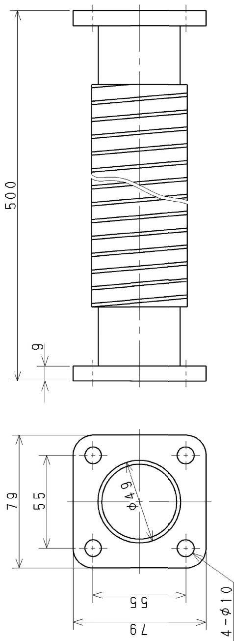
エキゾーストフレキ 1個
